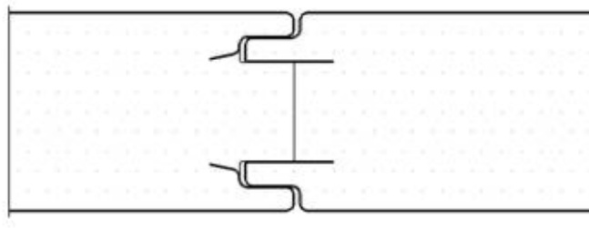
Строительная сэндвич-панель из профилированного листа (Рис. 1)
